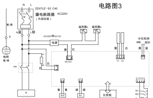
电路图3
