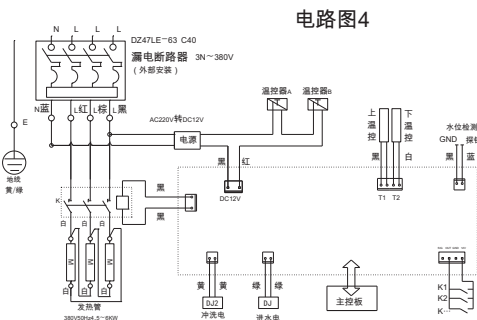
电路图4
